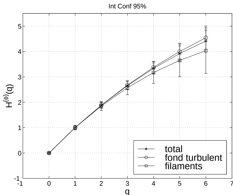
Fig. V.23: Fonctions H^{(\phi)}(q) pour l'ensemble, le fond turbulent et les filaments seuls dans le SF 6 ( H^{(\phi)}(1) = 1 par convention). Les trois estimations se confondent aux barres d'erreur près ( R_\lambda = 800 , dispositif n°2). Les barres d'erreur reflètent des intervalles de confiance à 95%.
